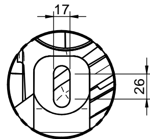
DETALLE B
