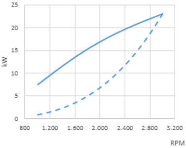
Potência (ISO 3046/1)
