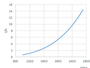
Potrošnja goriva
