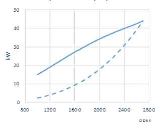
Puissance (ISO 3046/1)
