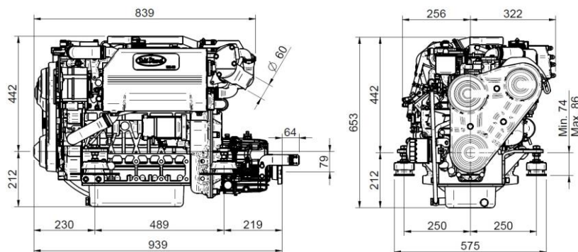
Moteur SK-60 Inv.TMC-60P 2,00:1
