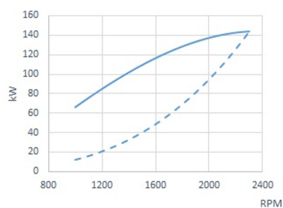
Effekt. Enligt ISO 3046/1
