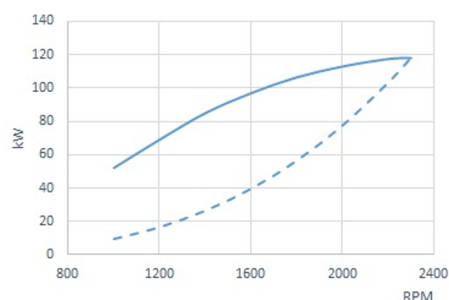
Moć. Prema ISO 3046/1
