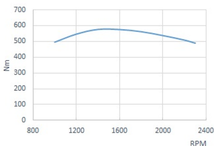
Okretni moment na radilici
