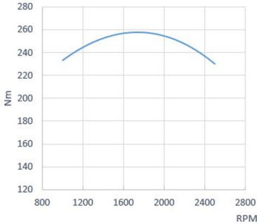
Par de motor da cambota
