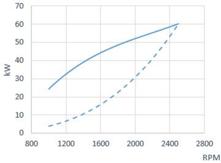
Potência (ISO 3046/1)
