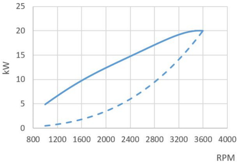
Potência (ISO 3046/1)
