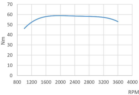
Par de motor da cambota
