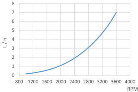
Consumo de combustível
