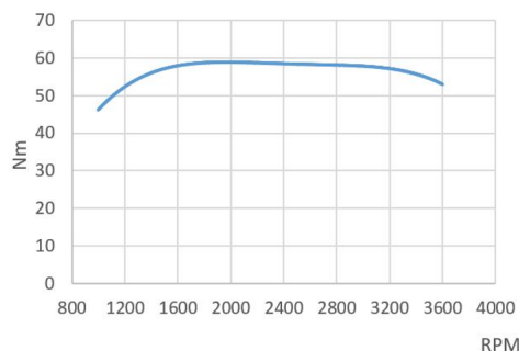
Okretni moment na radilici
