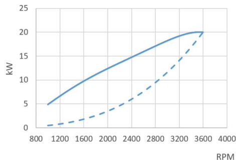
Moć. Prema ISO 3046/1
