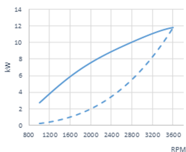
Effekt. Enligt ISO 3046/1
