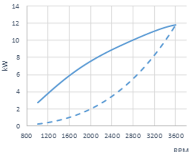
Potência (ISO 3046/1)
