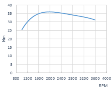
Okretni moment na radilici
