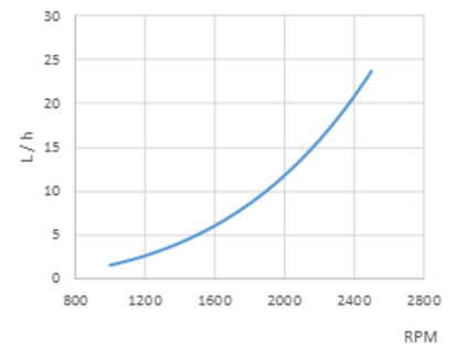
Brandstofverbruik
